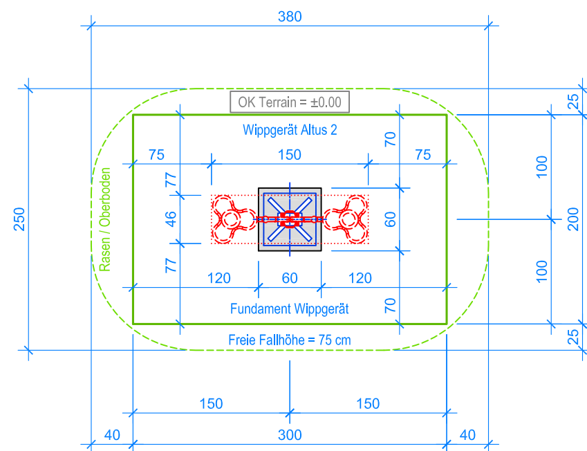
GRUNDRISS 1:50
