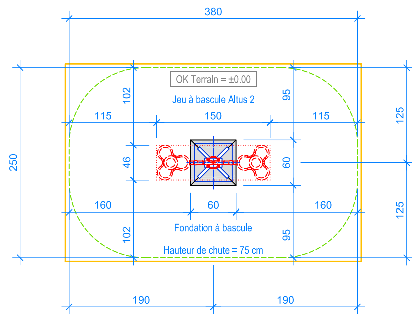
PLAN 1:50
