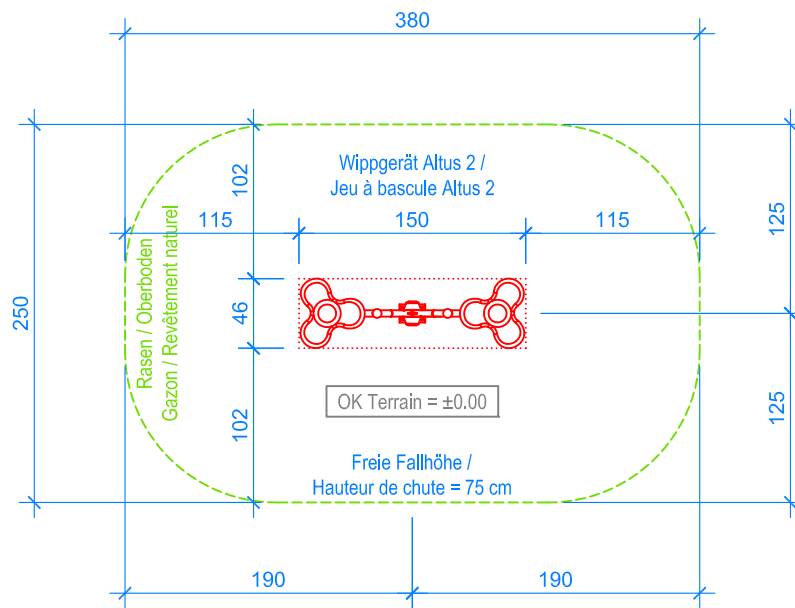
GRUNDRISS / PLAN 1:50
