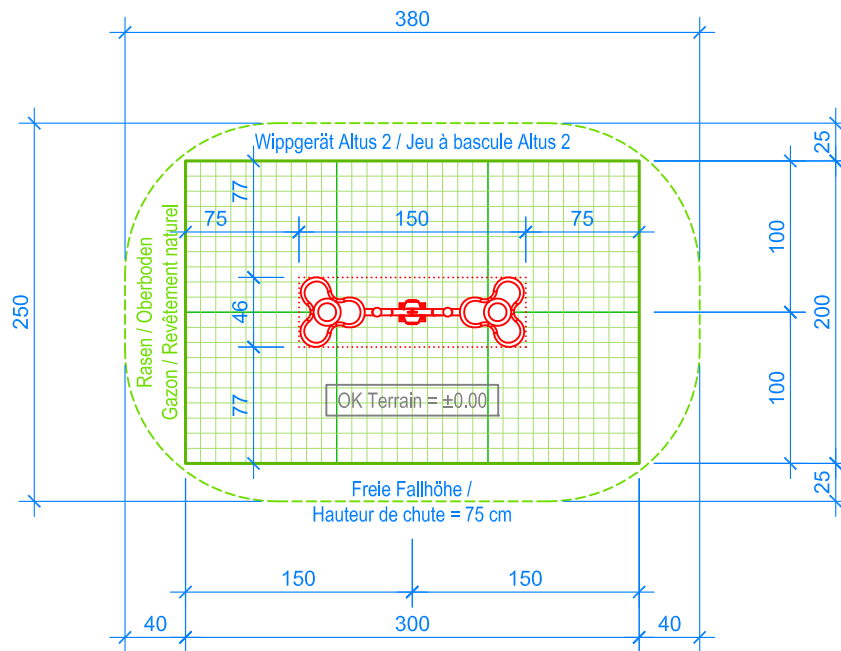
GRUNDRISS / PLAN 1:50
