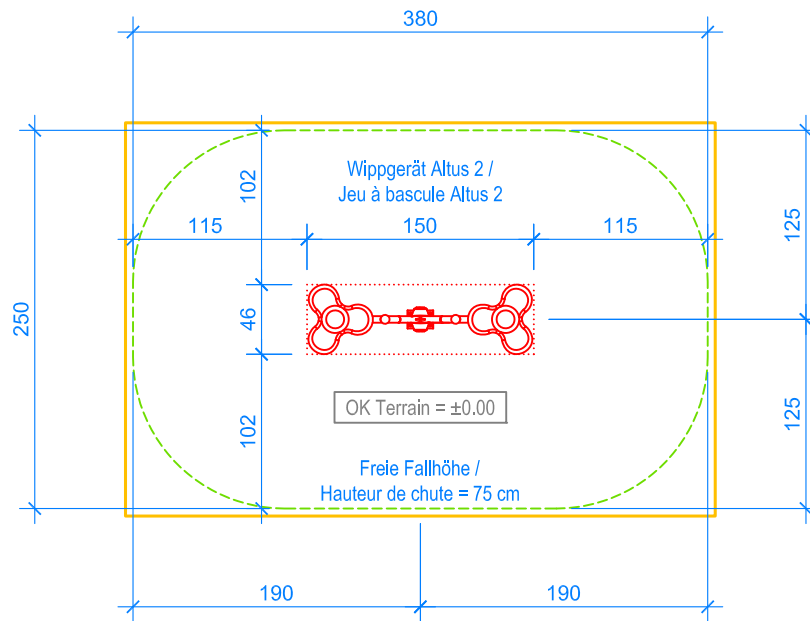
GRUNDRISS / PLAN 1:50
