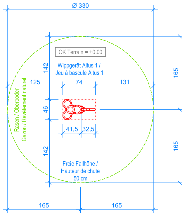
GRUNDRISS / PLAN 1:50
