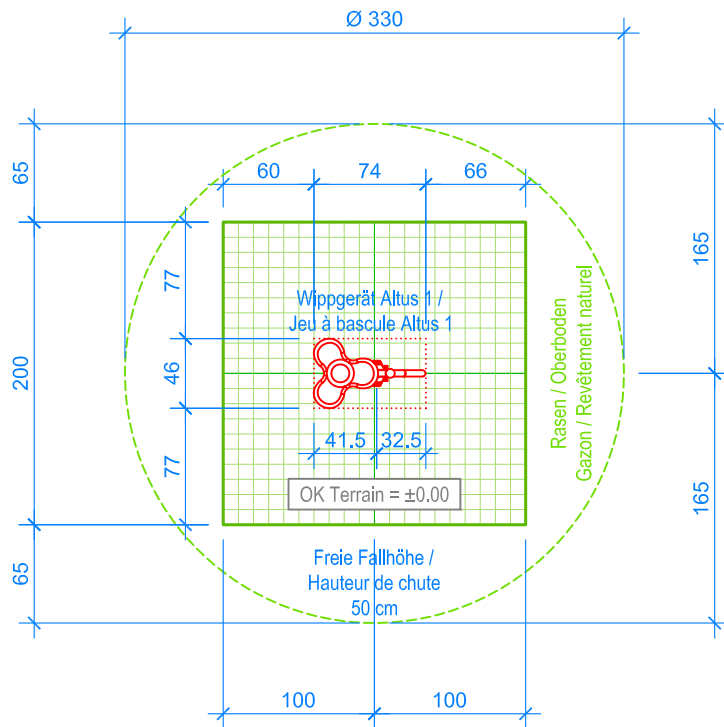
GRUNDRISS / PLAN 1:50
