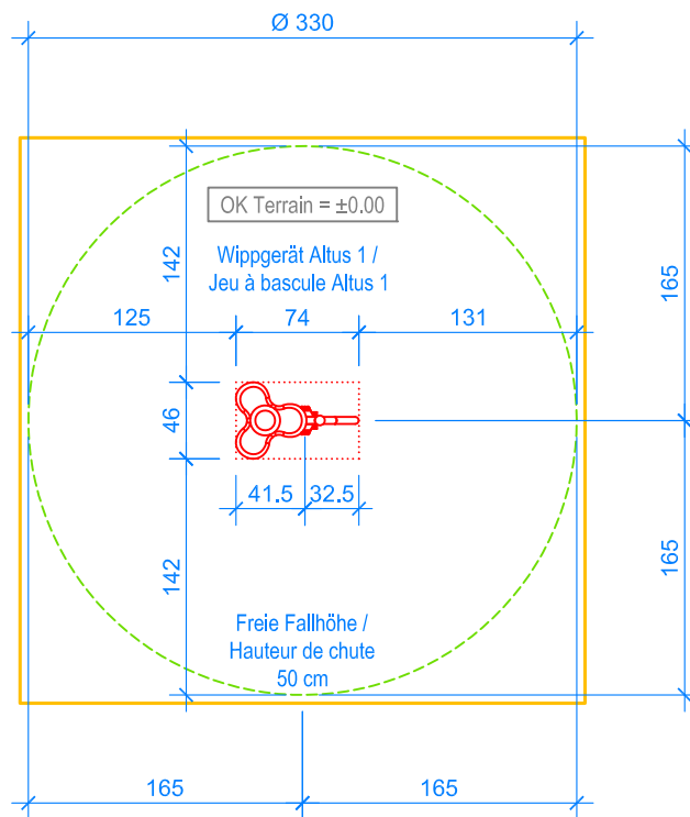
GRUNDRISS / PLAN 1:50
