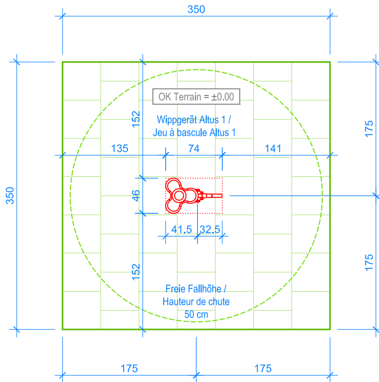
GRUNDRISS / PLAN 1:50
