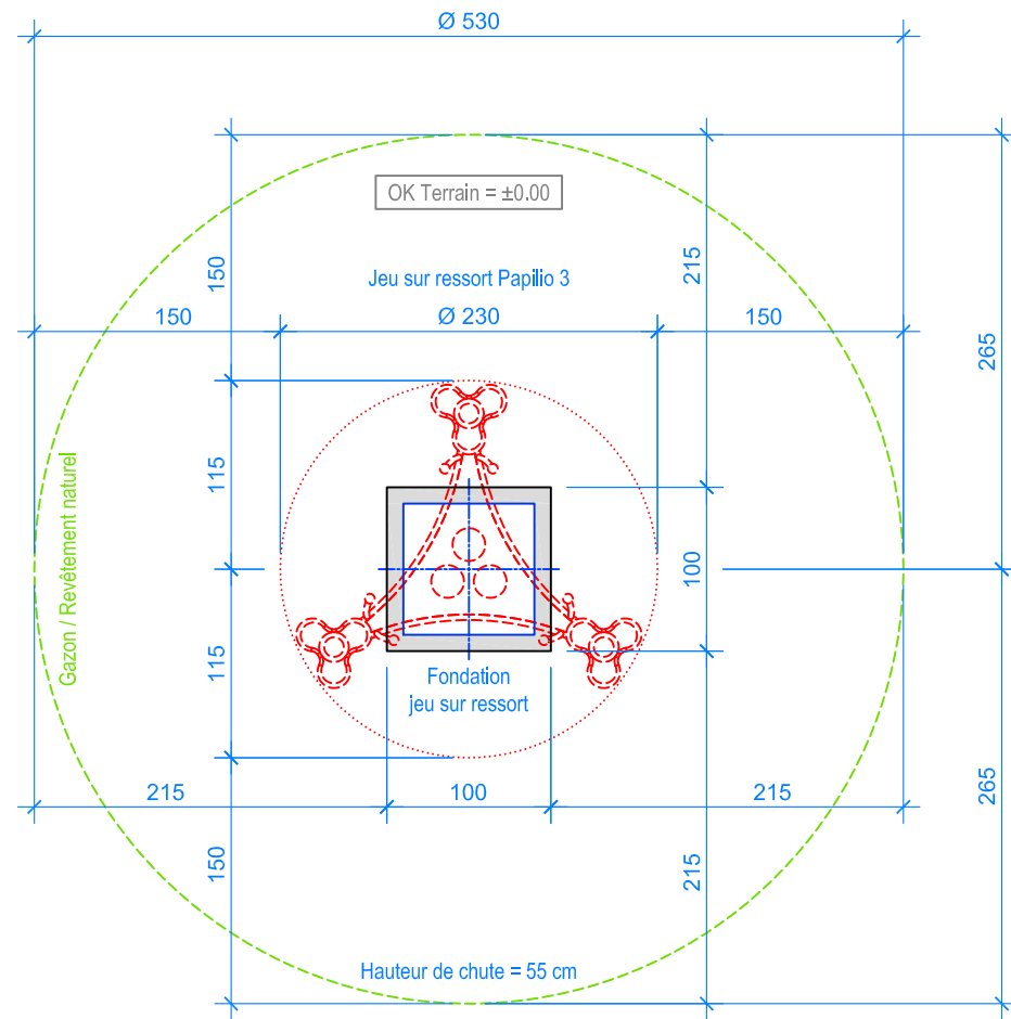
PLAN 1:50
