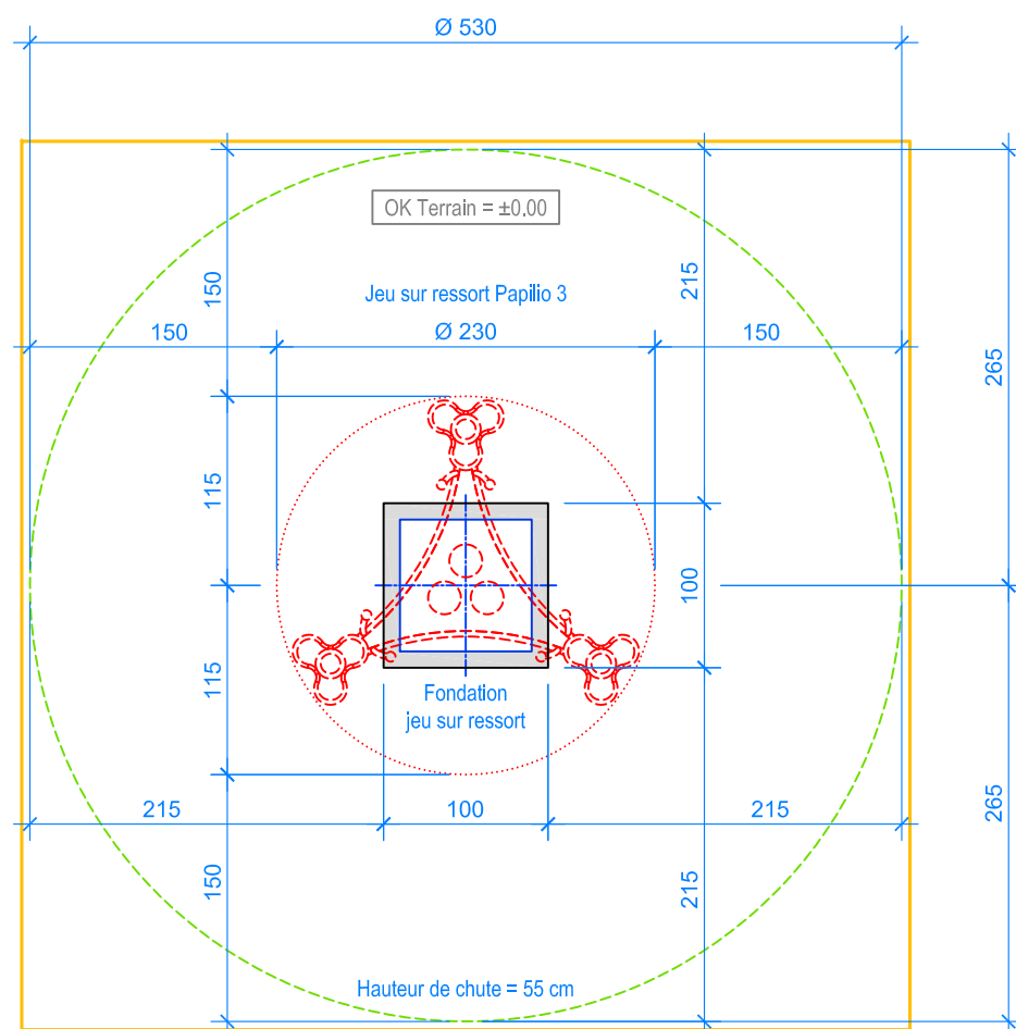
PLAN 1:50
