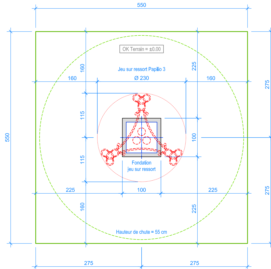
PLAN 1:50
