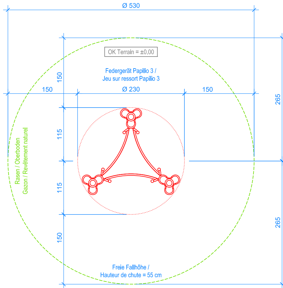
GRUNDRISS / PLAN 1:50
