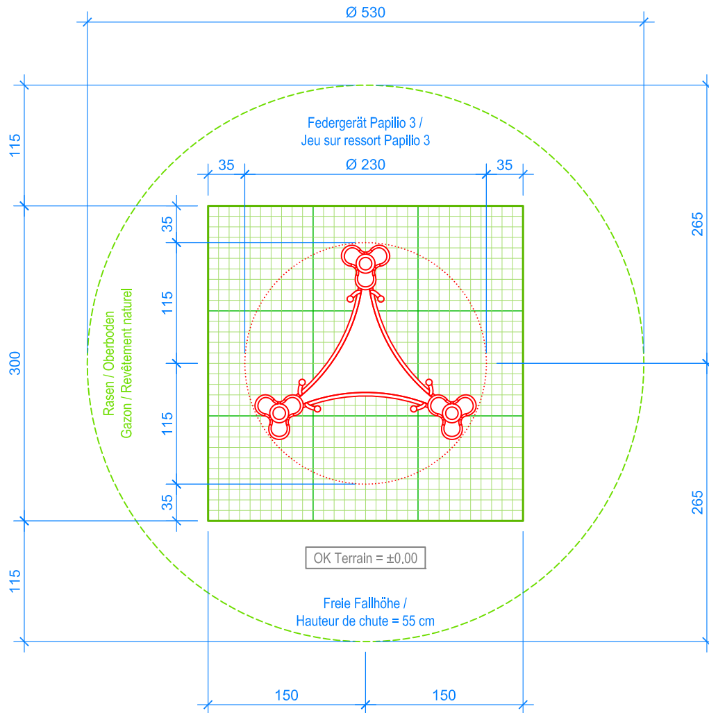
GRUNDRISS / PLAN 1:50
