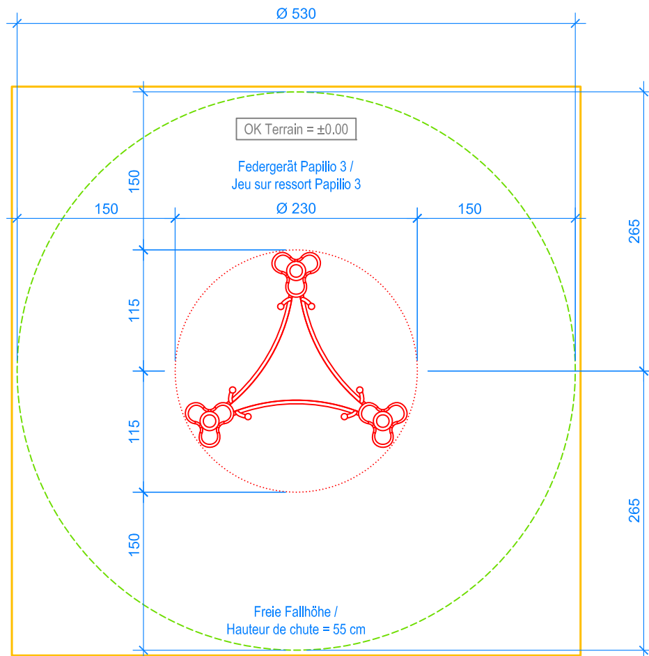
GRUNDRISS / PLAN 1:50
