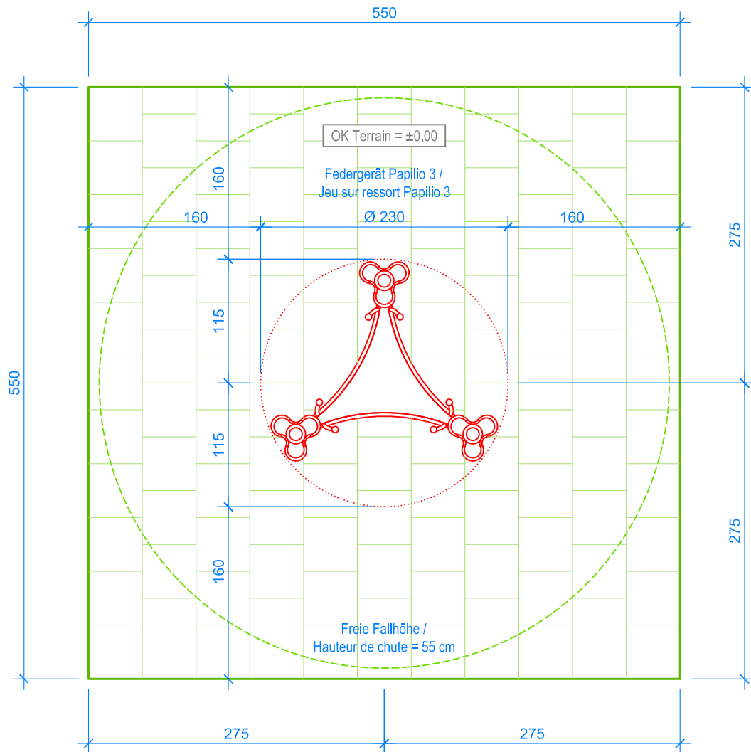
GRUNDRISS / PLAN 1:50
