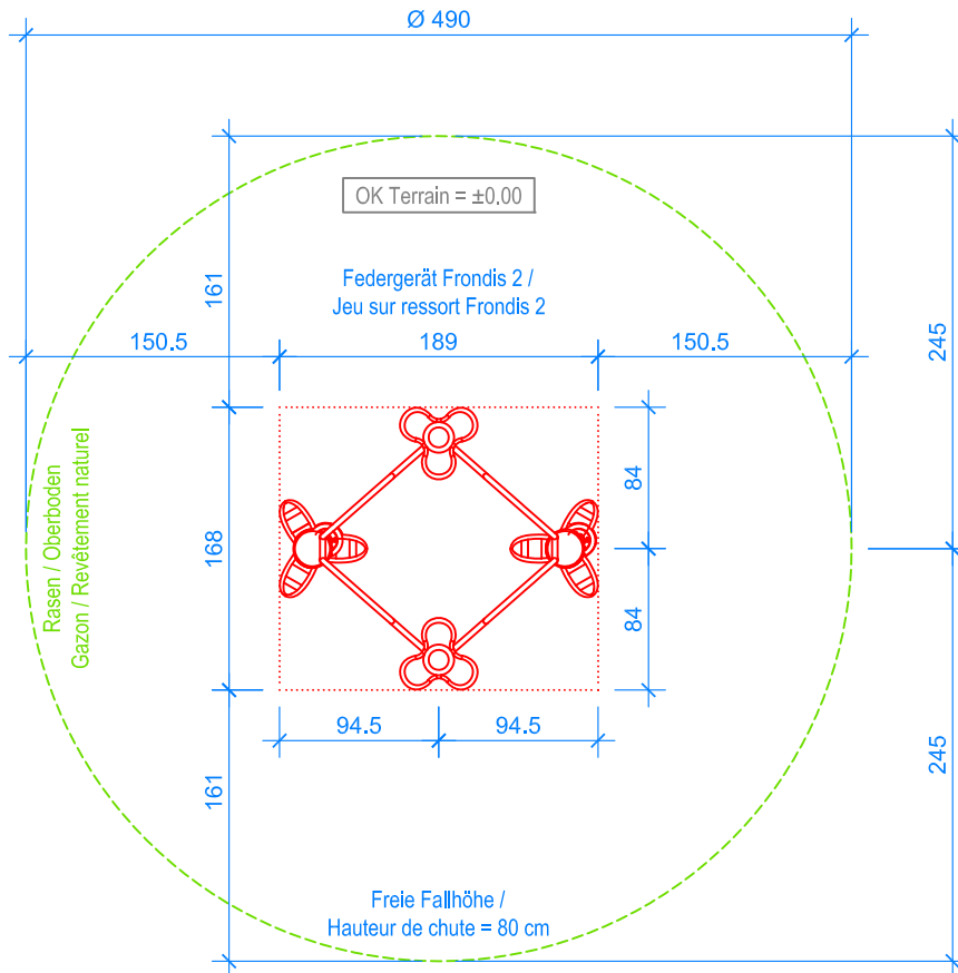
GRUNDRISS / PLAN 1:50
