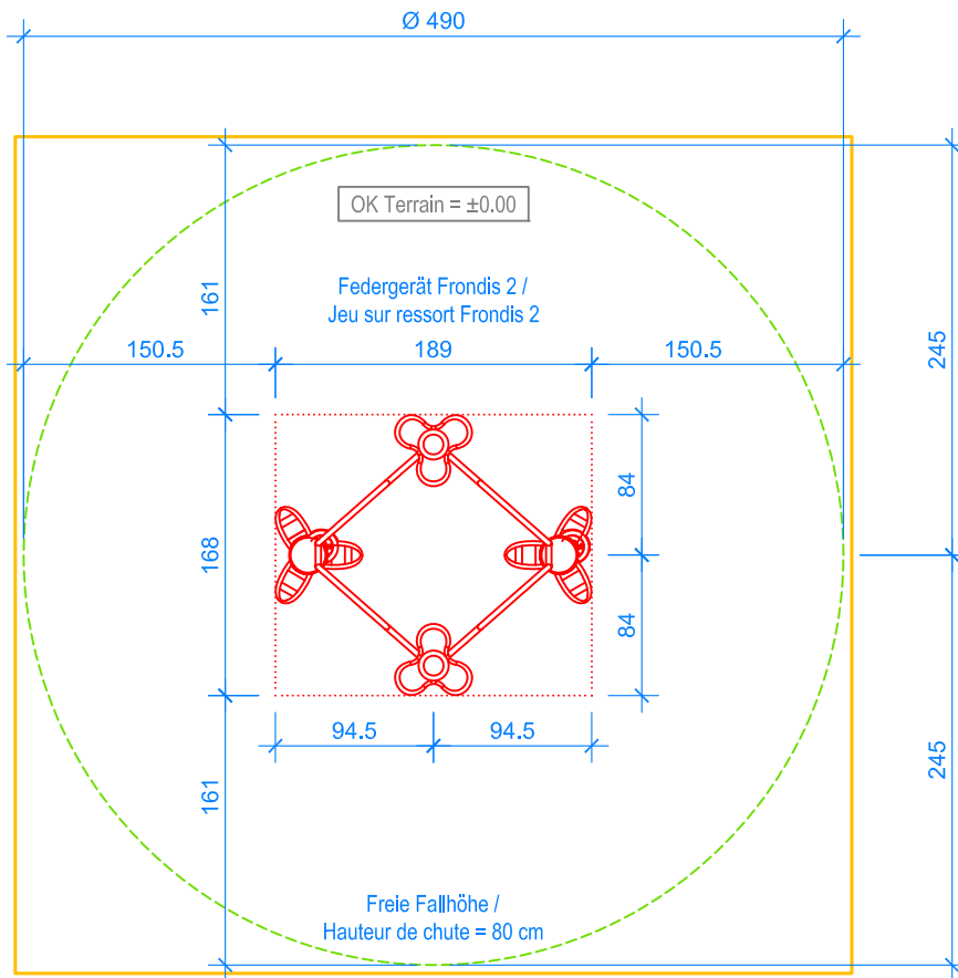
GRUNDRISS / PLAN 1:50
