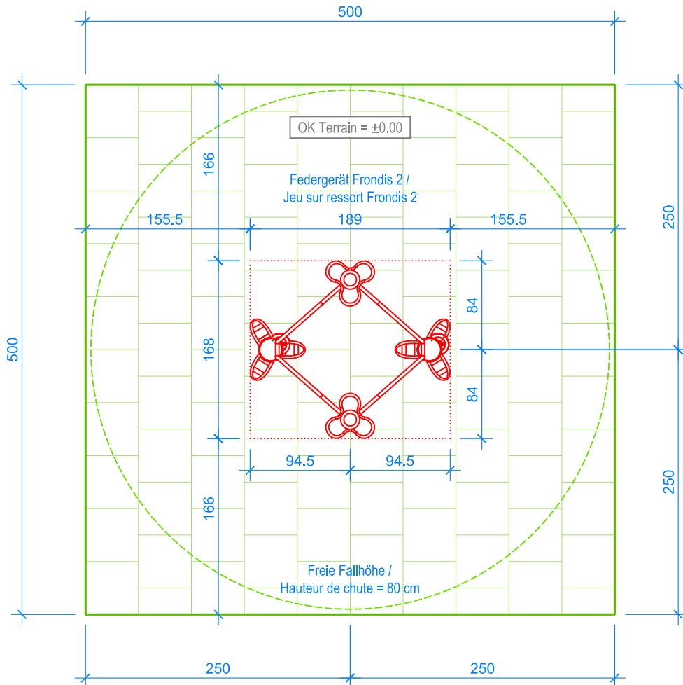
GRUNDRISS / PLAN 1:50
