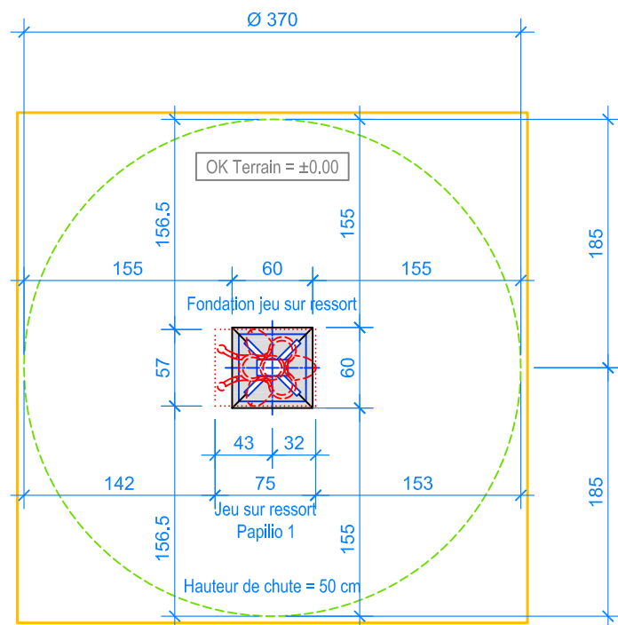
PLAN 1:50
