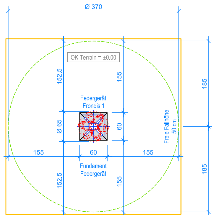
GRUNDRISS 1:50
