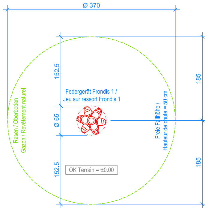
GRUNDRISS / PLAN 1:50
