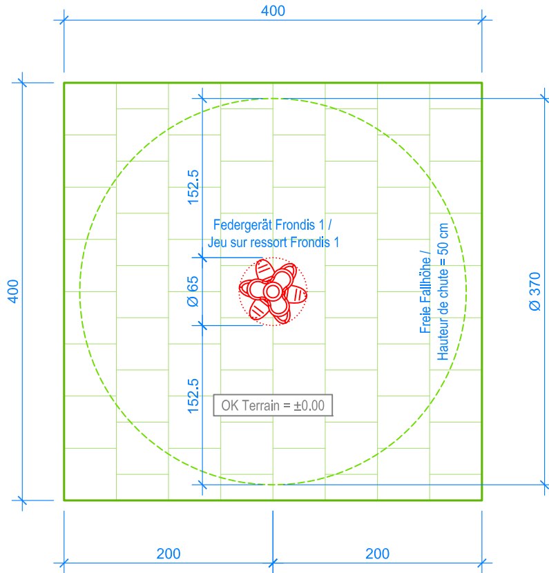
GRUNDRISS / PLAN 1:50
