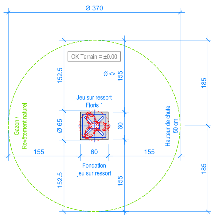
PLAN 1:50
