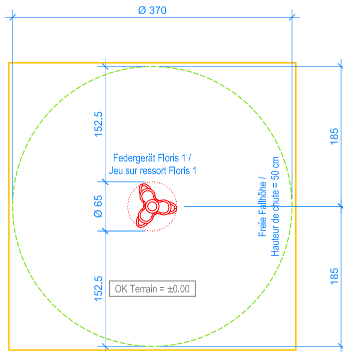
GRUNDRISS / PLAN 1:50
