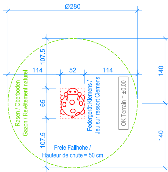
GRUNDRISS / PLAN 1:50
