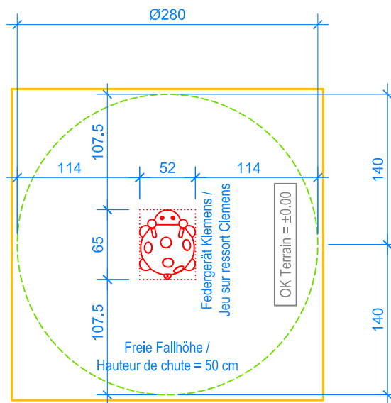
GRUNDRISS / PLAN 1:50
