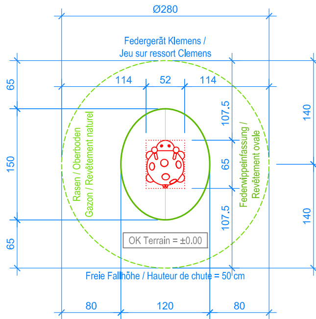
GRUNDRISS / PLAN 1:50
