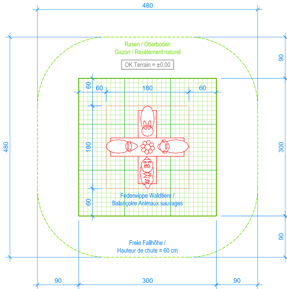
GRUNDRISS / PLAN 1:50
