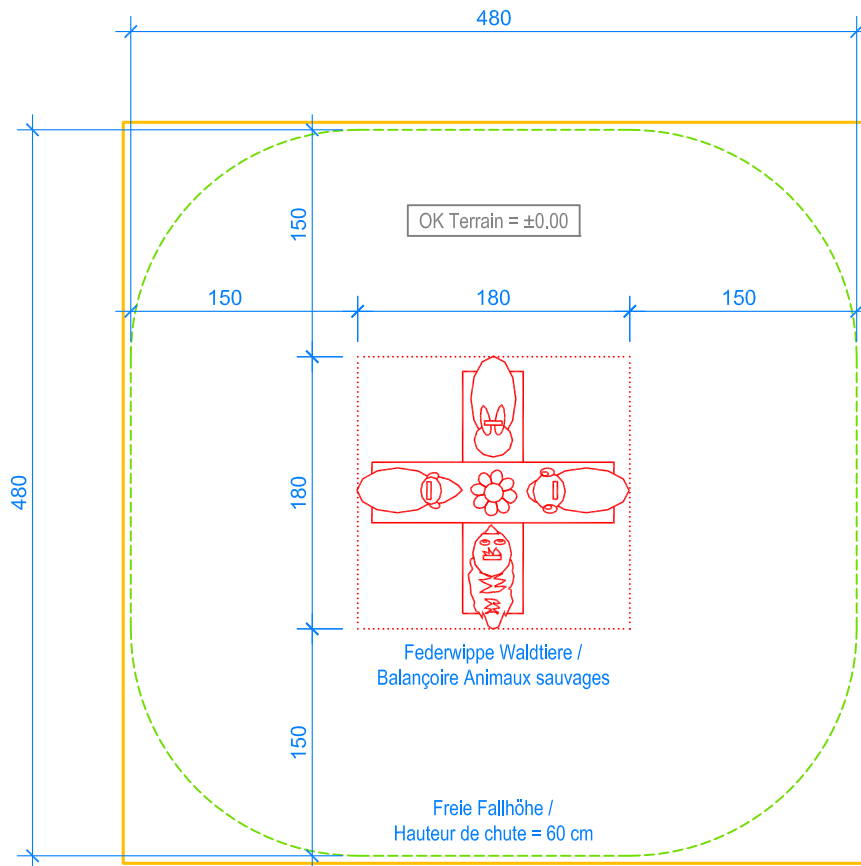
GRUNDRISS / PLAN 1:50
