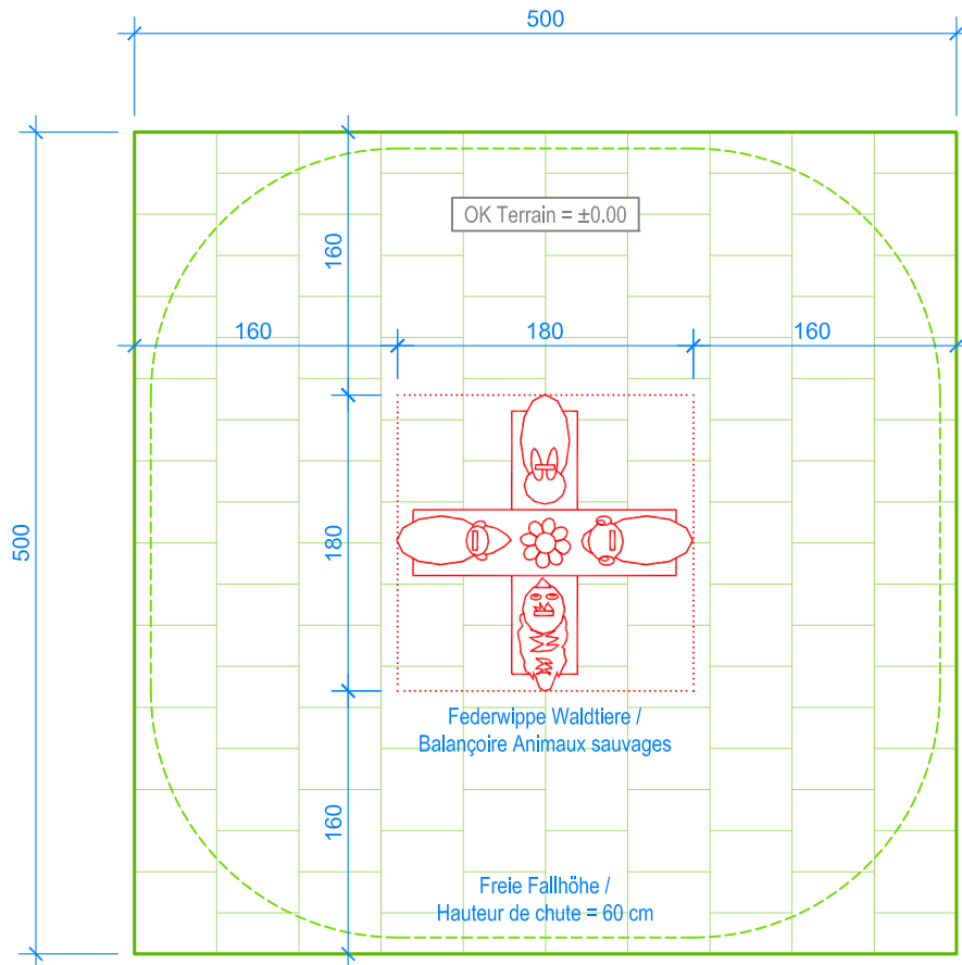
GRUNDRISS / PLAN 1:50
