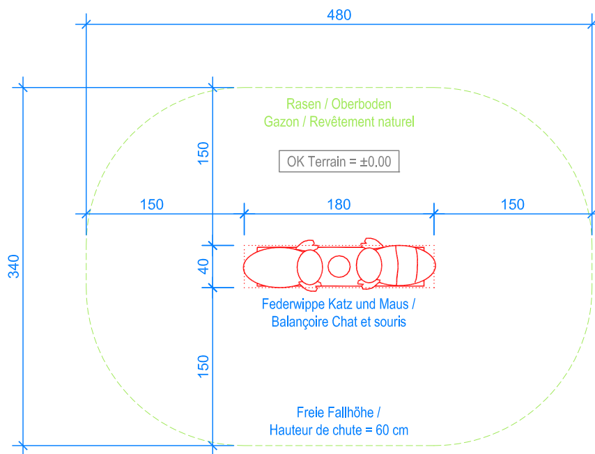
GRUNDRISS / PLAN 1:50
