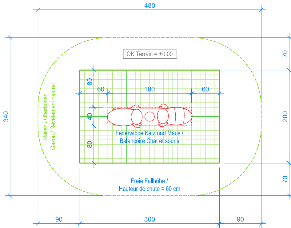
GRUNDRISS / PLAN 1:50
