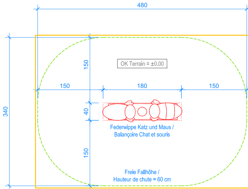
GRUNDRISS / PLAN 1:50
