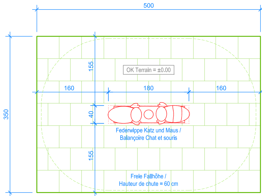
GRUNDRISS / PLAN 1:50
