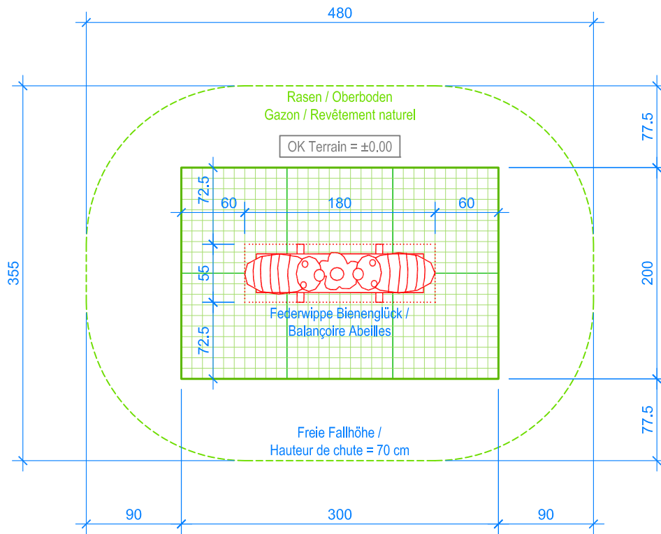
GRUNDRISS / PLAN 1:50
