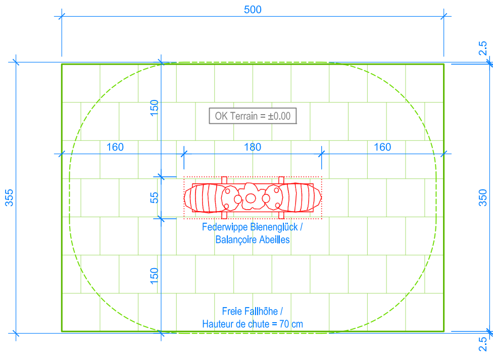
GRUNDRISS / PLAN 1:50
