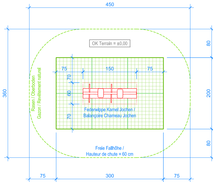
GRUNDRISS / PLAN 1:50
