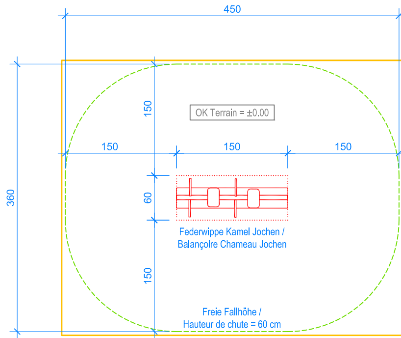
GRUNDRISS / PLAN 1:50
