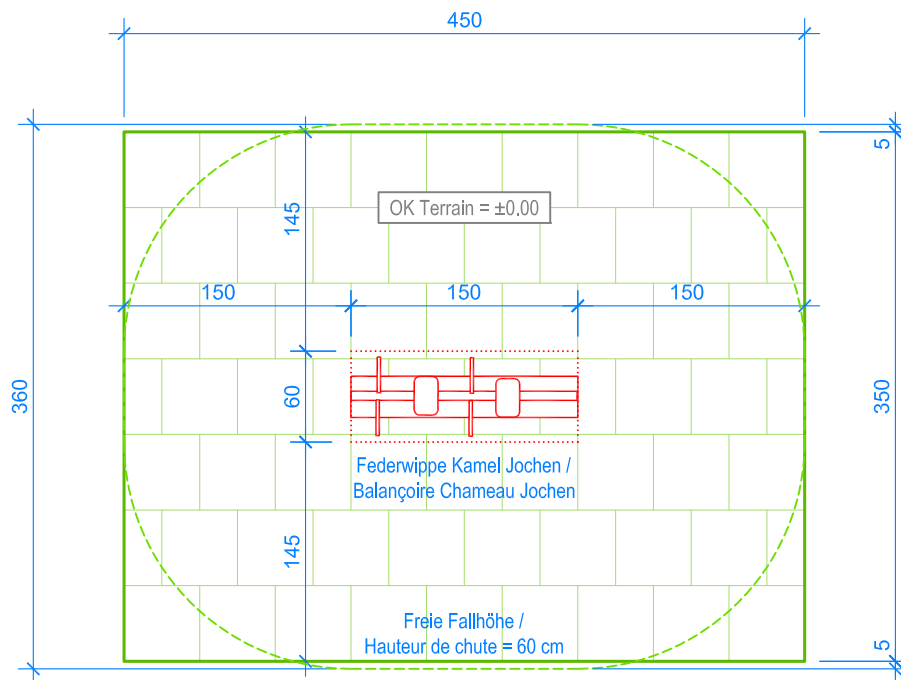
GRUNDRISS / PLAN 1:50
