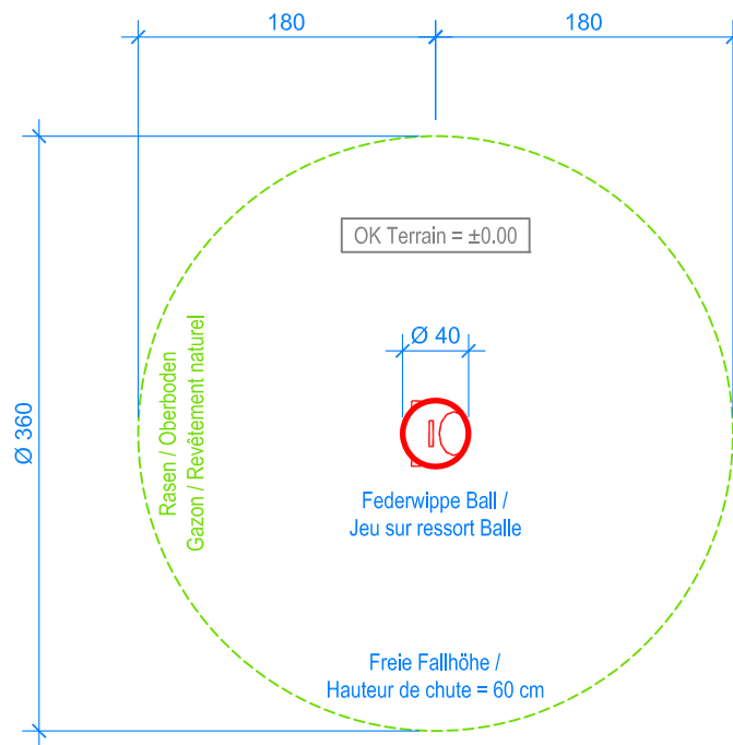
GRUNDRISS / PLAN 1:50
