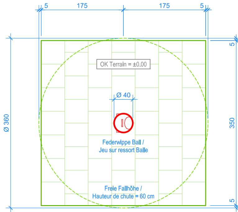
GRUNDRISS / PLAN 1:50
