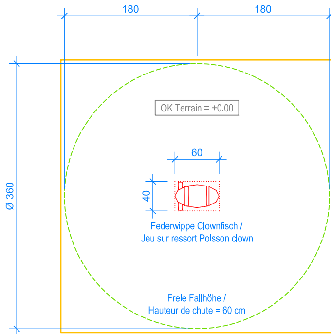
GRUNDRISS / PLAN 1:50
