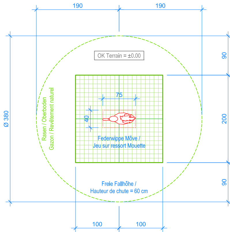
GRUNDRISS / PLAN 1:50
