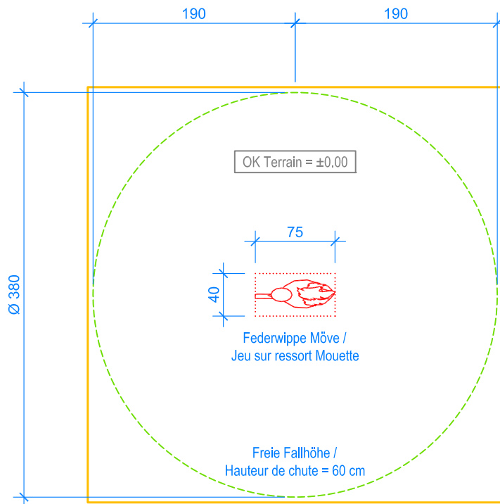
GRUNDRISS / PLAN 1:50
