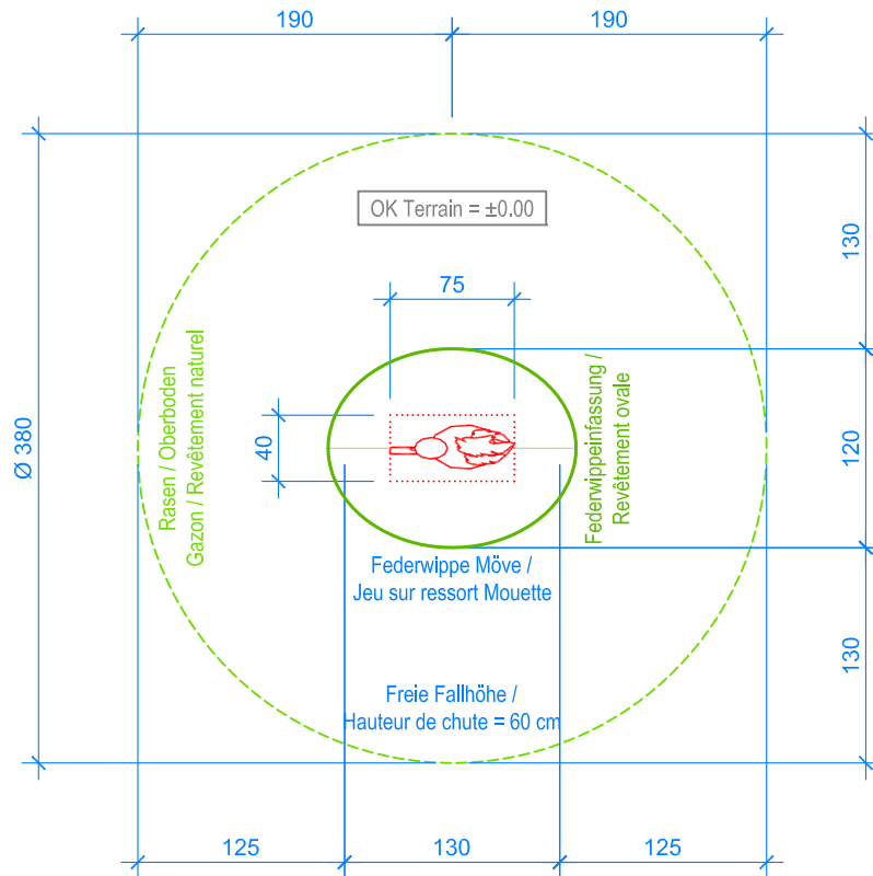
GRUNDRISS / PLAN 1:50
