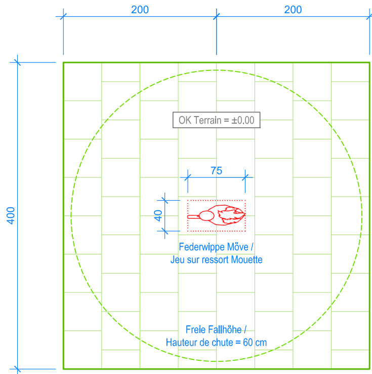
GRUNDRISS / PLAN 1:50
