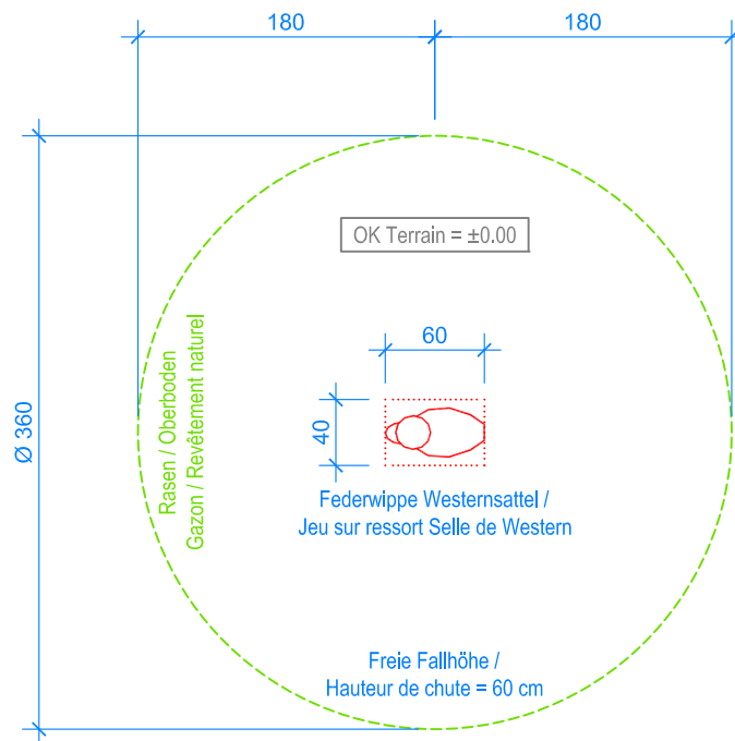
GRUNDRISS / PLAN 1:50
