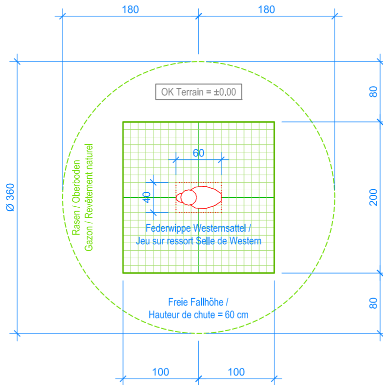
GRUNDRISS / PLAN 1:50
