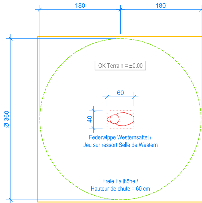
GRUNDRISS / PLAN 1:50
